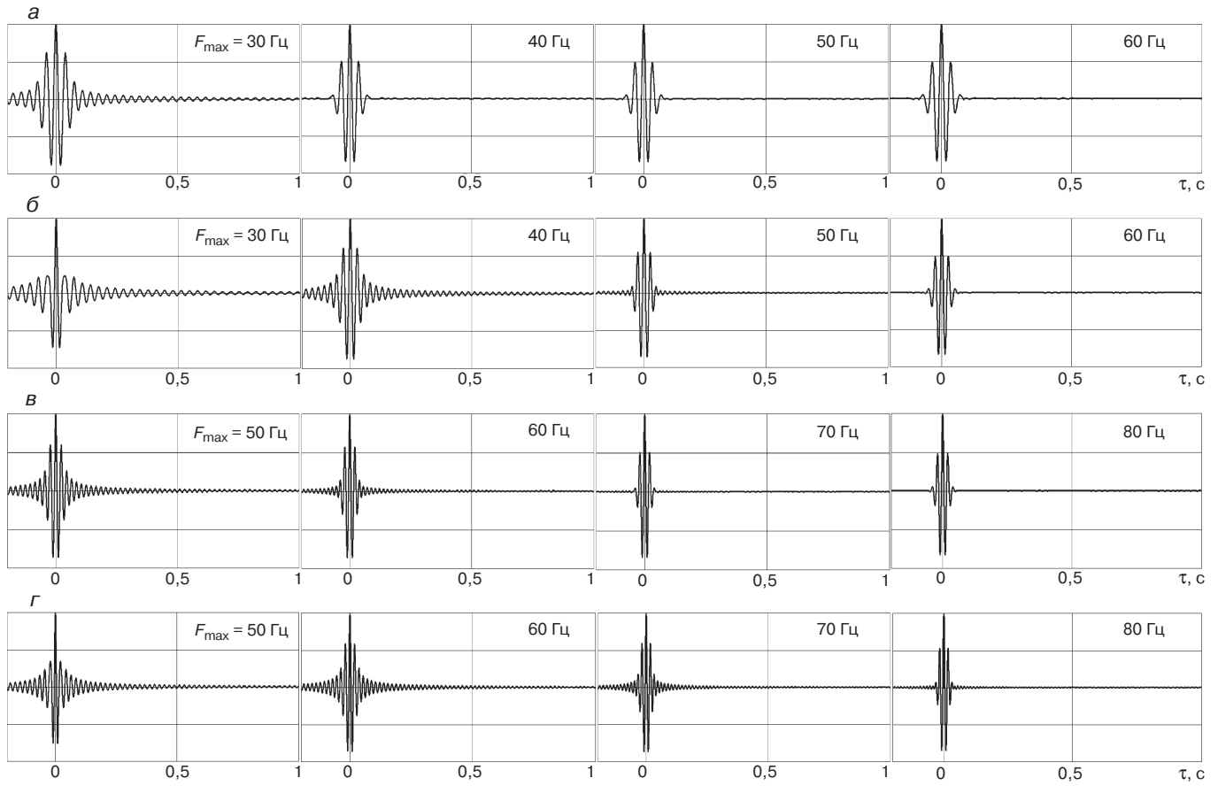
Рис. 2. Зависимость формы главного максимума ФVK последовательностей ЛИЧ от значений F_{\max} и f_{\text{вид}} : а - f_{\text{вид}} = 25 Гц; б - 35 Гц; в - 45 Гц; г - 55 Гц
