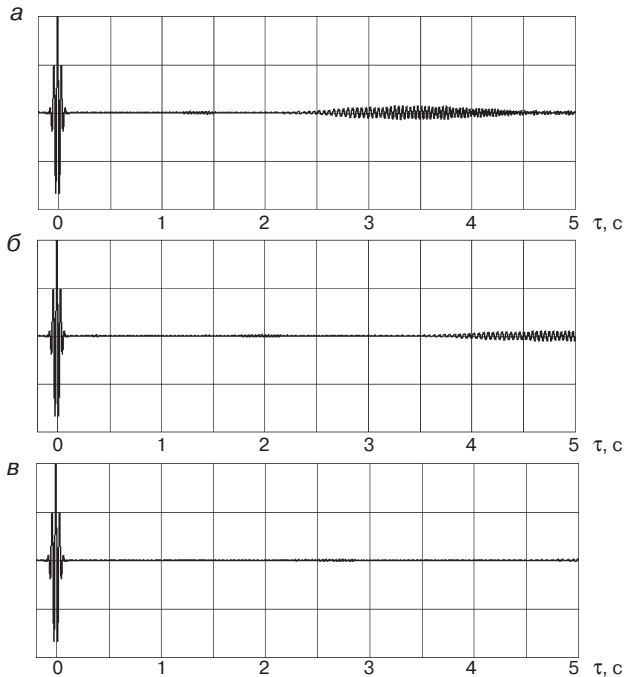
Рис. 3. ФVK последовательностей ЛИЧ при различных значениях T ( f_{\text{вид}} = 25 Гц; \Delta f 10 - 50 Гц): а - T = 10 с; б - T = 15 с; в - T = 20 с
