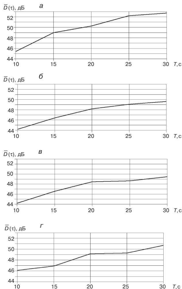
Рис. 4. Средние значения \bar{D}(t) в интервале от 0,5 с до t_H в зависимости от T :
